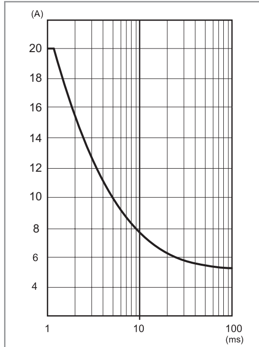
P782E-1 Pico de corriente de salida en función del tiempo (78.2E)
