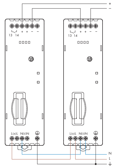
Conexión en serie
