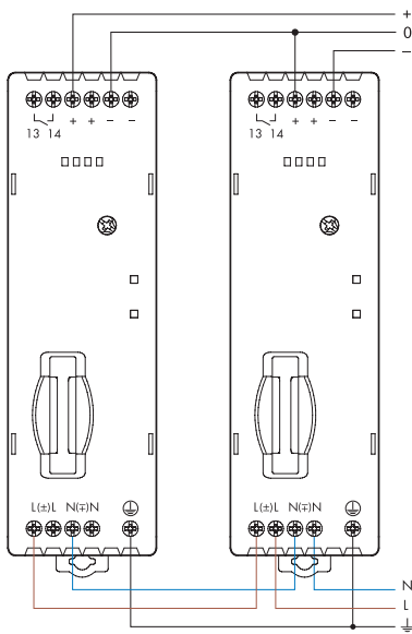
Conexión dual
