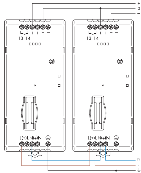
Conexión dual
