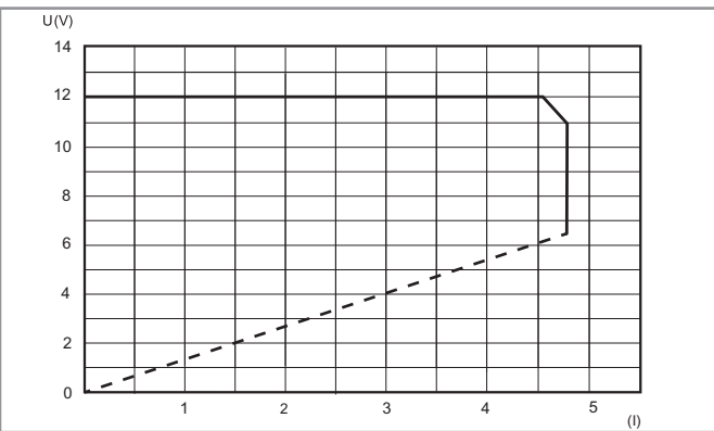
FB78-3 Tensión de salida en función de la corriente de salida (78.1C)
