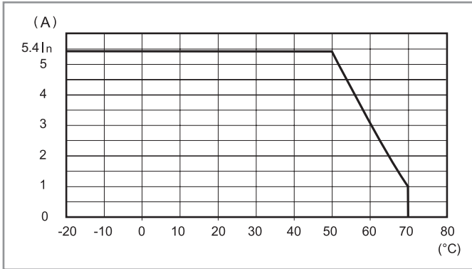
L78-8 Corriente de salida en función de la temperatura ambiente (78.1D)
