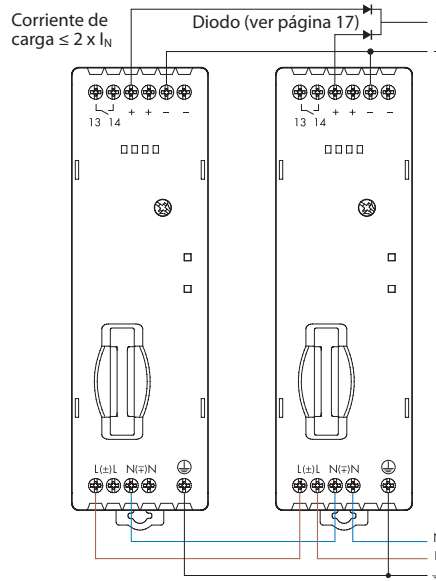
Conexión en paralelo
