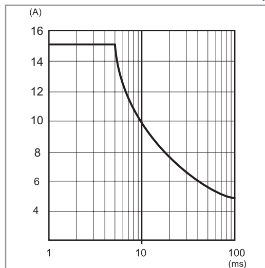
P78-7 Pico de corriente de salida en función del tiempo (78.1C)
