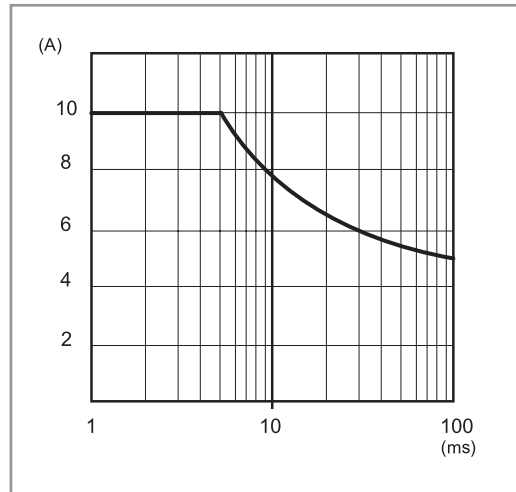
P78-7 Pico de corriente de salida en función del tiempo (78.1C)
