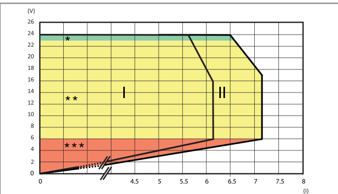
FB78-3 Tensión de salida en función de la corriente de salida (78.1C)
