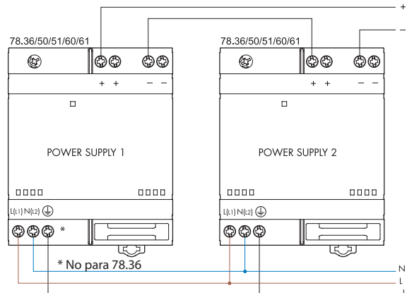
Conexión en serie
