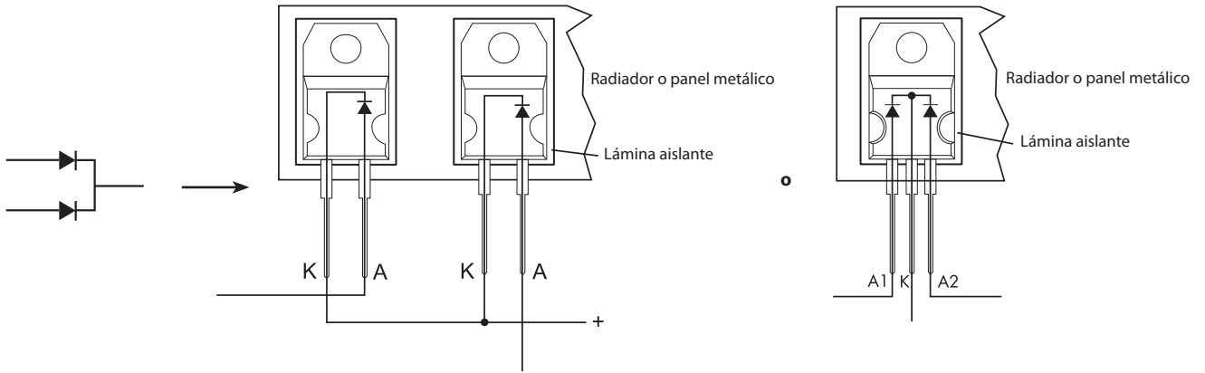
Diodo para los tipos 78.36, 78.50, 78.60, 78.51, 78.61
