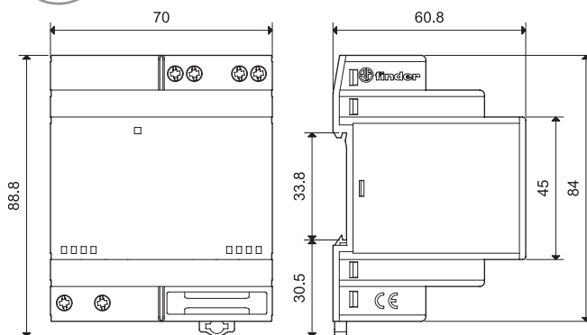
78.51 / 78.61 Borne de jaula
