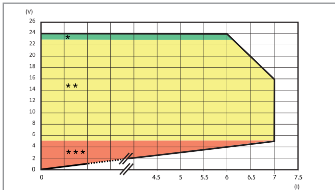
FB78-4 Tensión de salida en función de la corriente de salida (78.1D)
