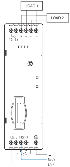
78.1D - Conexión de la fuente de alimentación
