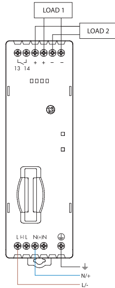
Conexiones básicas 78.1C - Conexión de la fuente de alimentación
